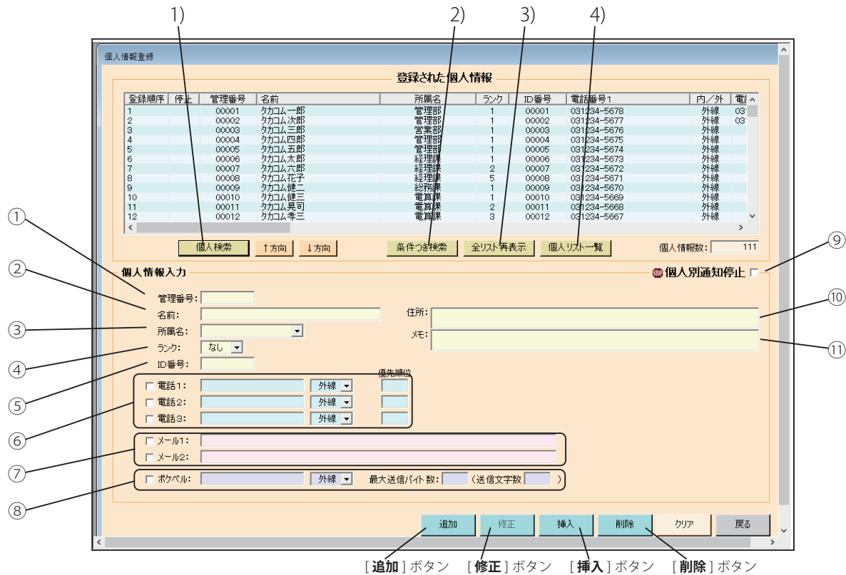
【「個人情報登録」画面】
