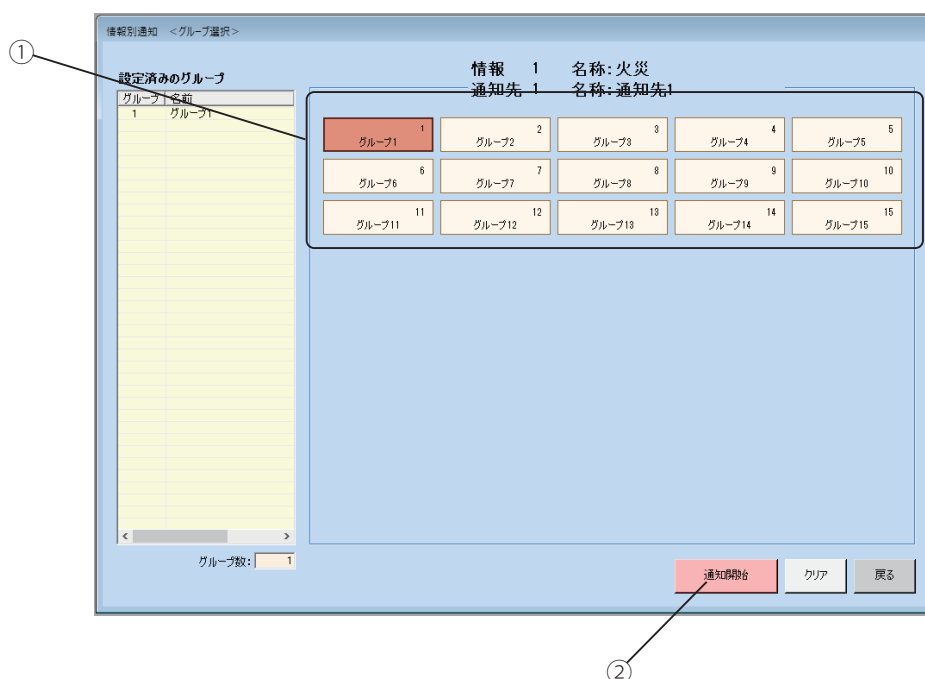
【「情報別通知＜グループ選択＞」画面】
