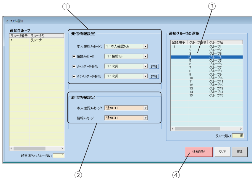
【「マニュアル通知」画面】
