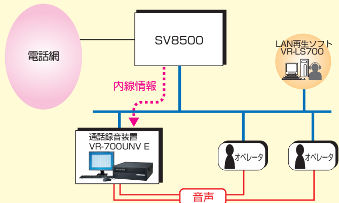
VR-700UNV E 電話機接続の場合
