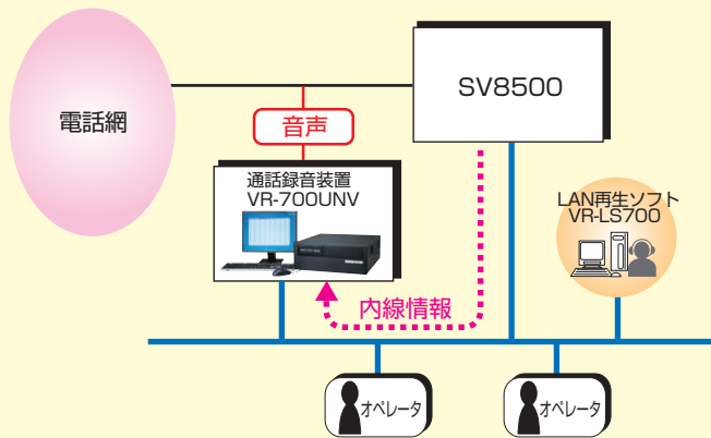
VR-700UNV 外線接続の場合
